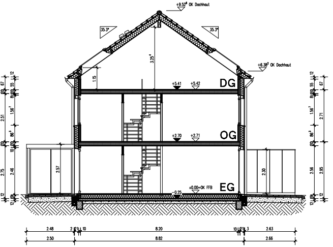
Schnitt
