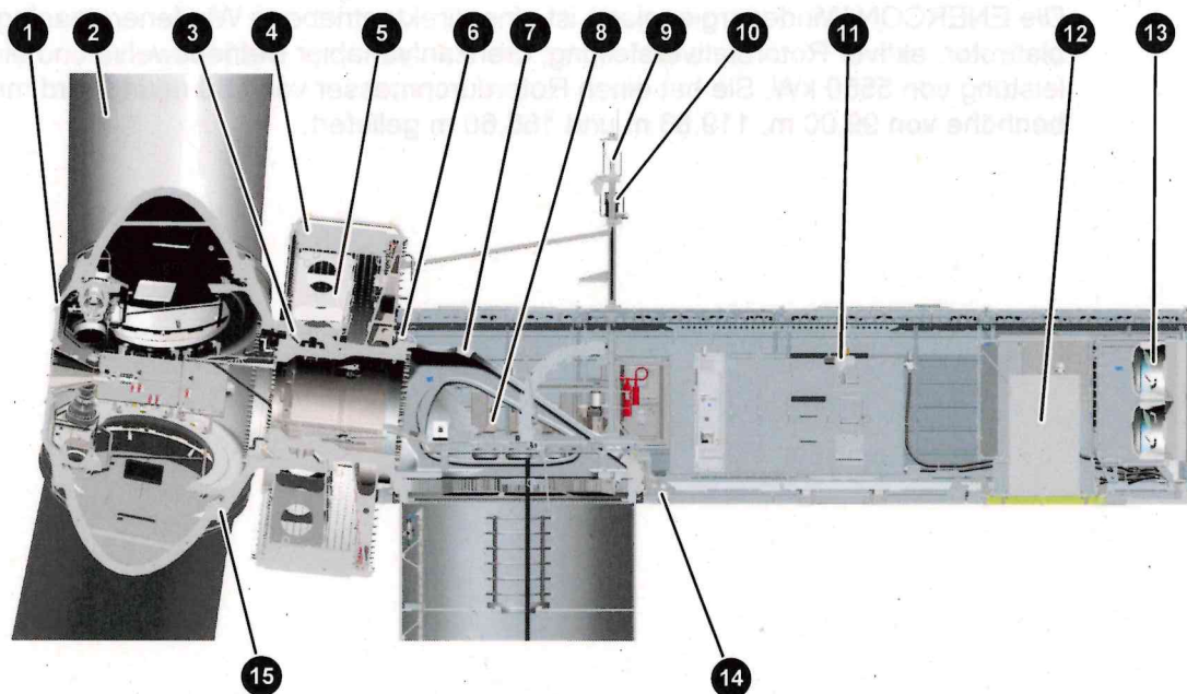
Abb. 1: Gondelschnitt
