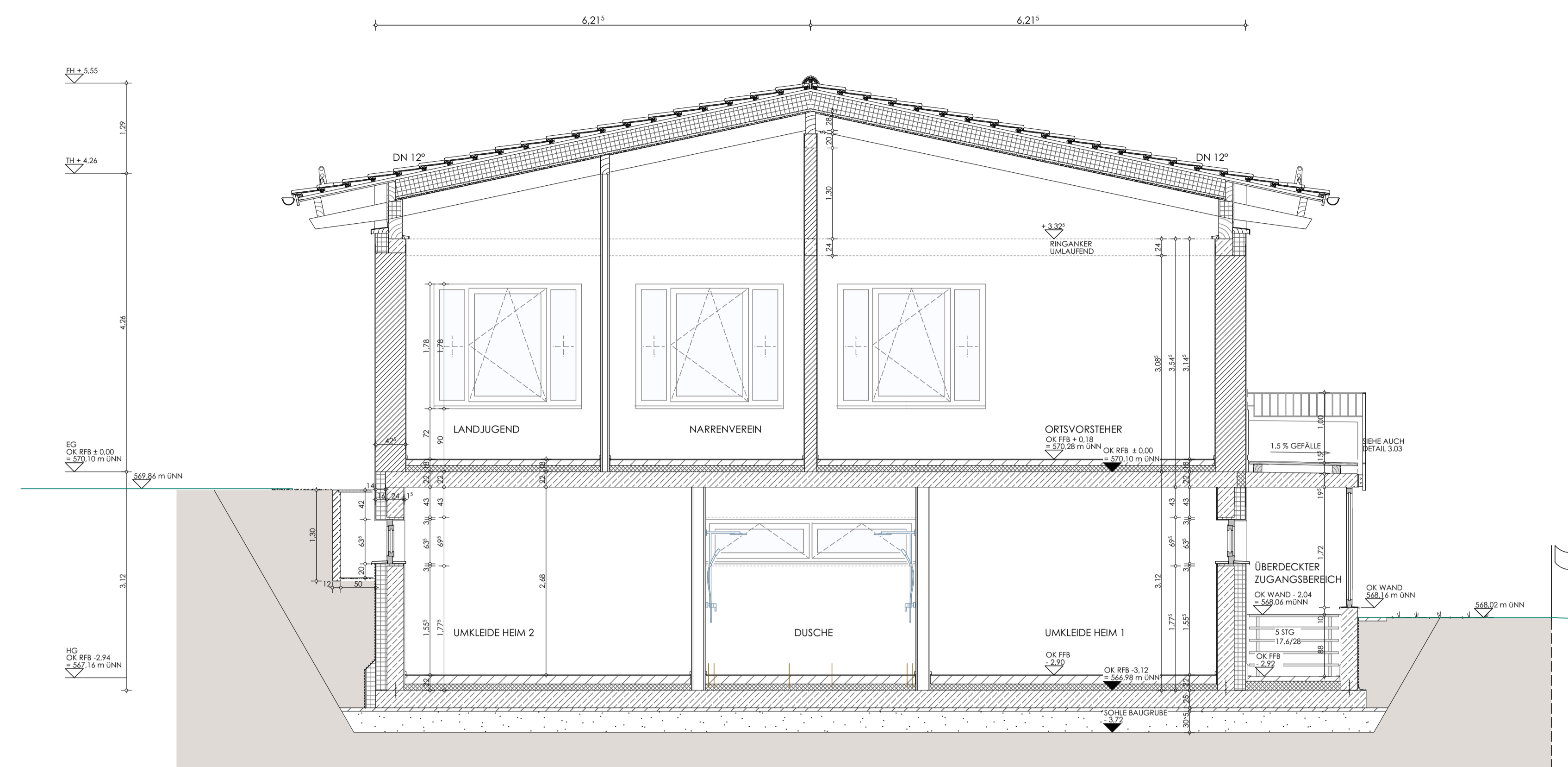
SCHNITT 2 - 2
