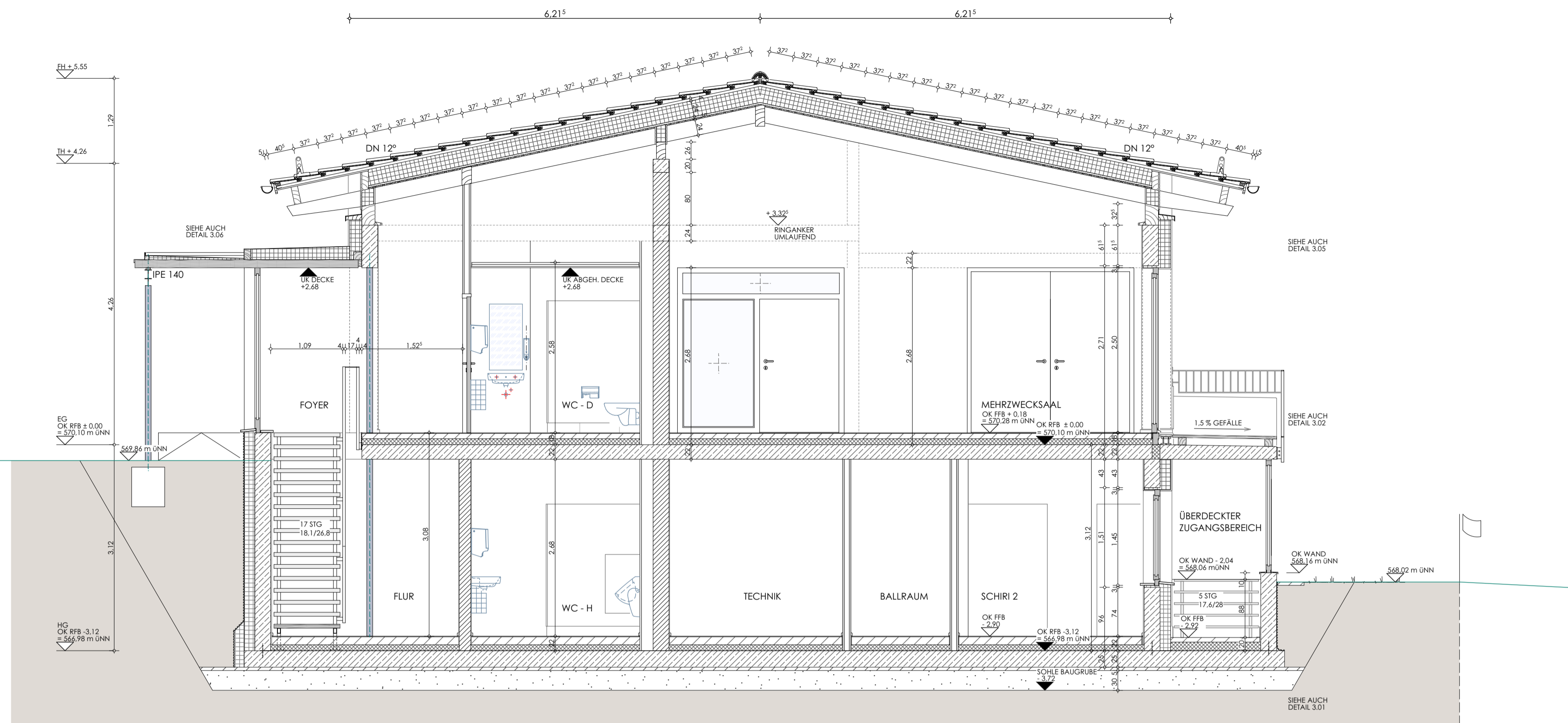
SCHNITT 1 - 1
