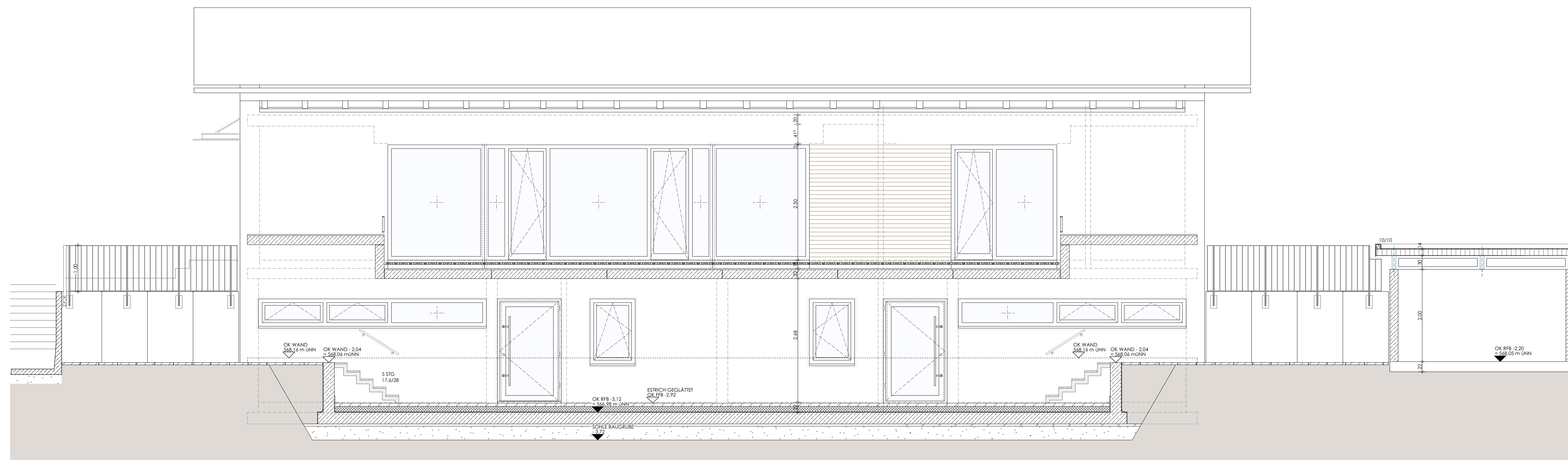
SCHNITT 3 - 3
